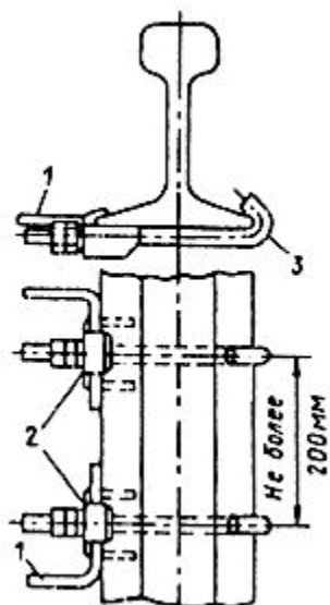
Рис. 3. Присоединение к тяговому рельсу проводников защитного заземления:
