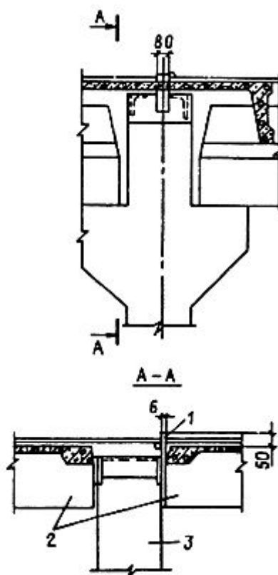
Рис. 24. Узел в системе молниезащиты многоэтажного здания с железобетонными ригелями с полками: 1 - соединительная деталь; 2 - плиты покрытия; 3 - колонна
