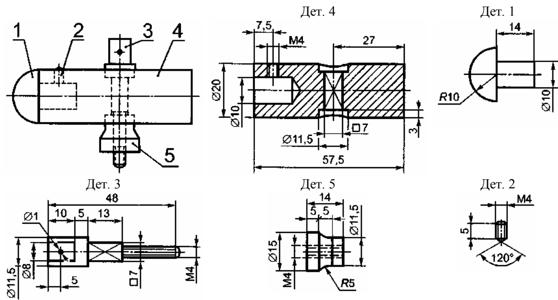
б — Ударный элемент маятникового молотка
